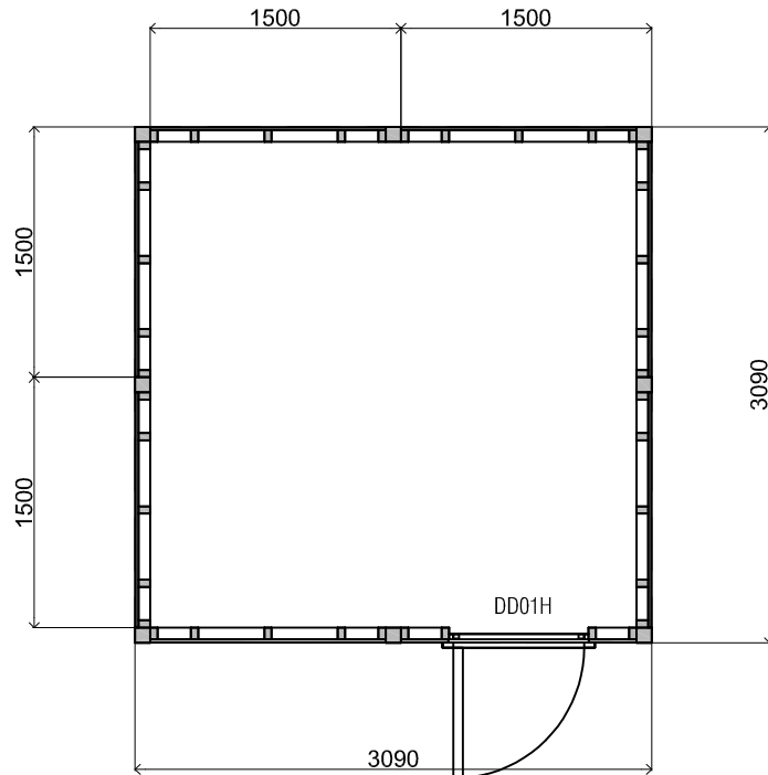
Plattegrond / Plan
